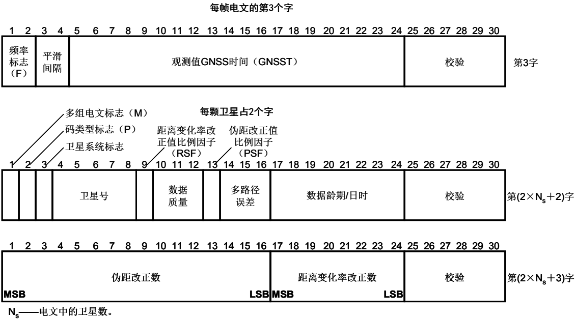
图 L.5 电文类型 21 的格式
