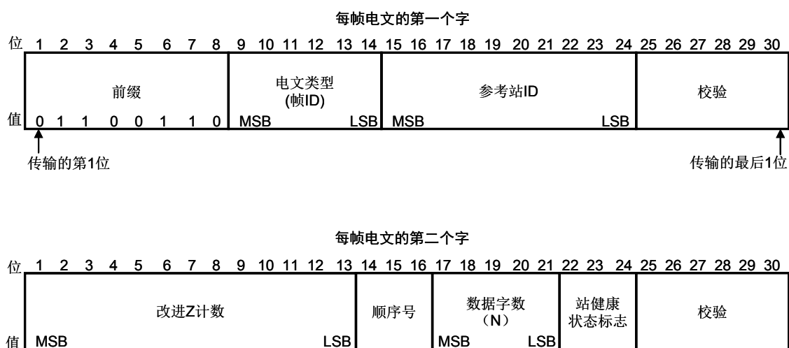
图 1 电文头格式
