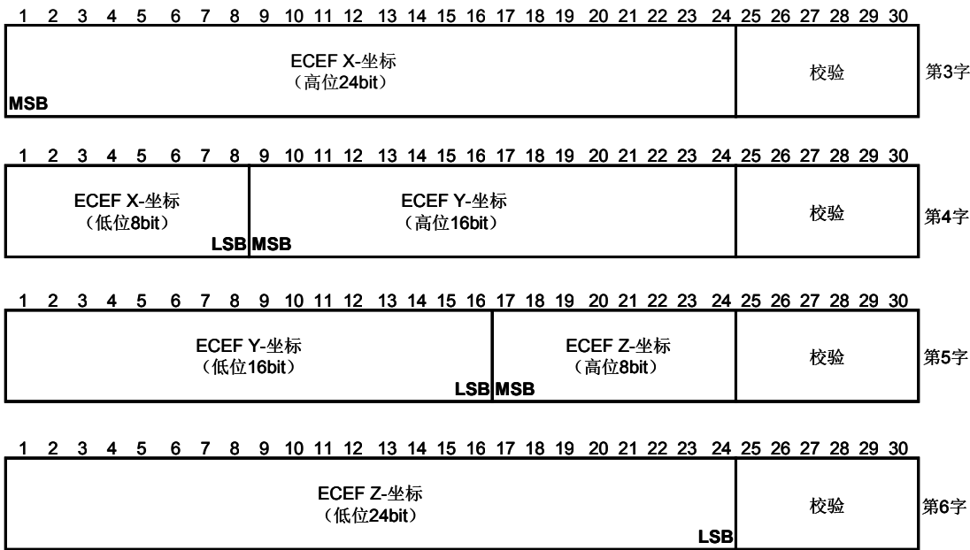
图 3 电文类型 3 的格式
