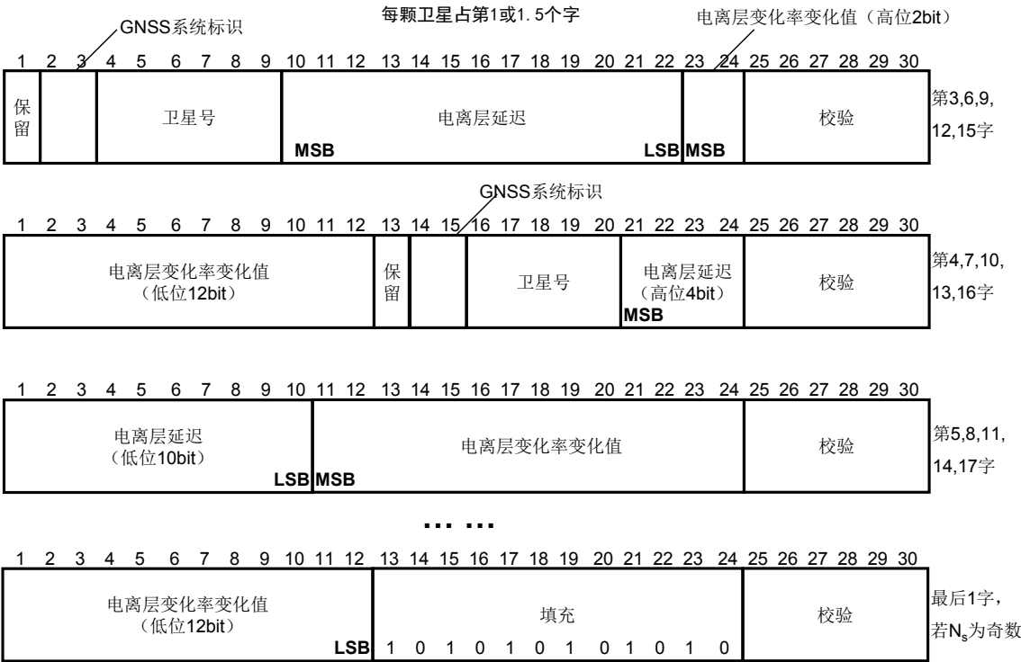
图 7 电文类型 15 的格式
