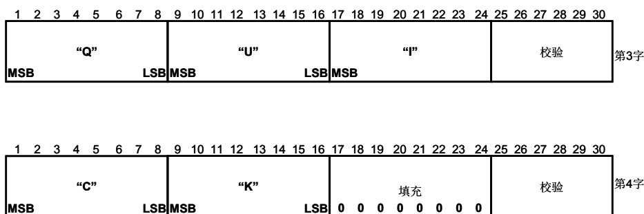
图 8 电文类型 16 的格式
