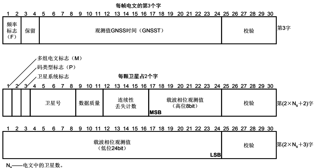
图 L.2 电文类型 18 的格式
