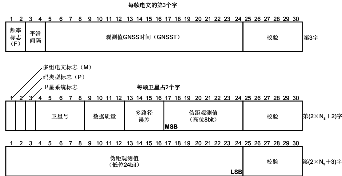
图 L.3 电文类型 19 的格式
