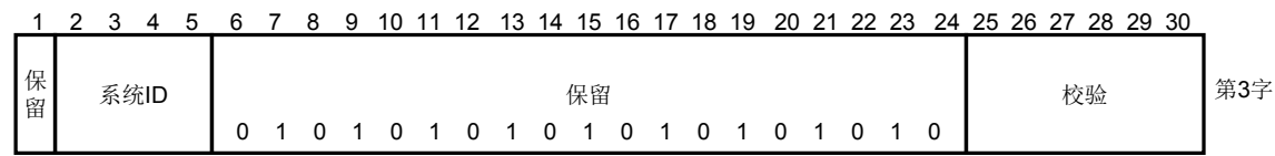
图 19 电文类型 42-GNSS 空帧
