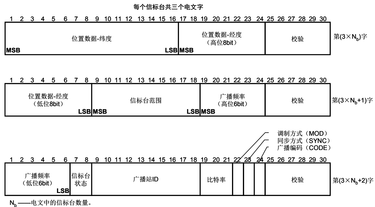
图 15 电文类型 35 的格式
