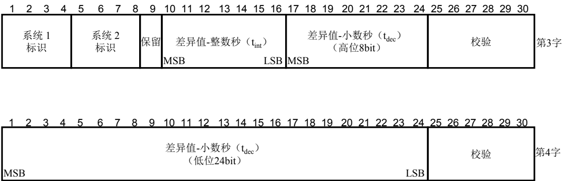
图 17 电文类型 37 的格式
