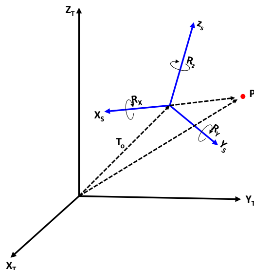
图 2 坐标系三维转换的平移和旋转
