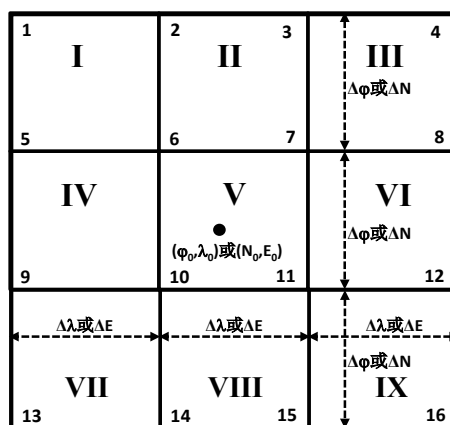
图 4 残差电文的格网定义
