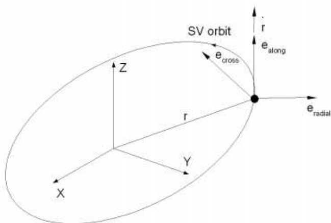
图 8 径向、切向、垂直轨迹方向的分量
